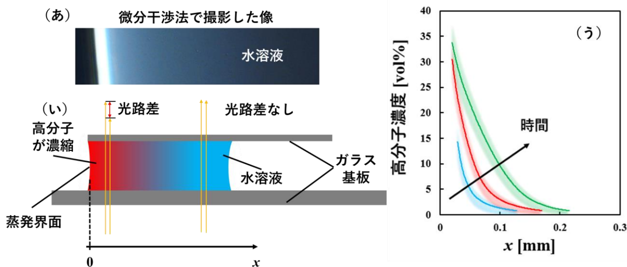
図 1 高分子溶液を微分干渉法で観察した透過像（あ）は、ガラスセル（い）を用いて撮影した。水の蒸発によって高分子が濃縮すると、ガラスセル内の溶液の位置によって光路長が変化する（（い）参照）。光路長が変化した位置では透過像の明るさが変わる。（あ）では、明るくなっている部分で高分子が濃縮され、濃度分布が付いている。この明るさの分布を検量線によって濃度分布に変換した（う）。グラフ（う）は、同じサンプルを異なる乾燥時間（青、赤、緑の順で乾燥時間が長い）で計測した結果を示す。乾燥時間が長くなるほど、高分子の濃度が高くなっている。グラフ（う）の横軸は、（い）の x 軸に対応する。
