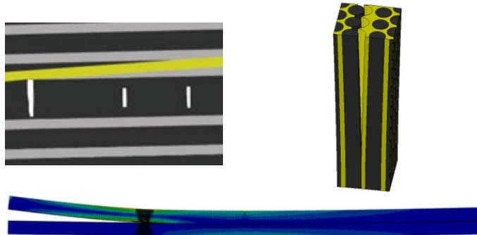
高精度数値解析技術の構築
