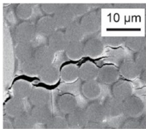
微視的リアルタイム損傷観察
