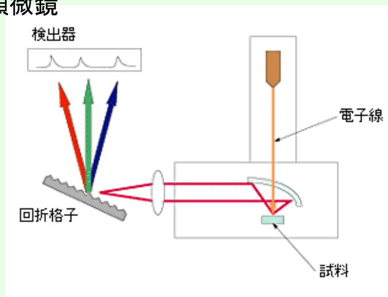
分光器
