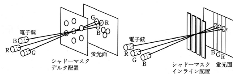
(b) カラーブラウン管の電子銃、シャドーマスク、蛍光体の配置
