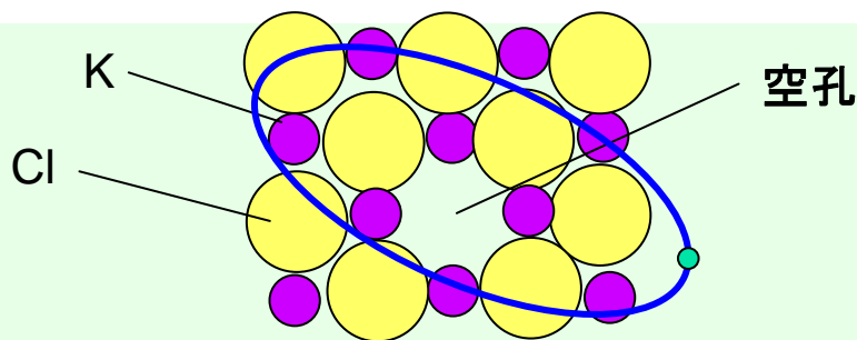
図4.35 KClのF中心の関与する発光と吸収
