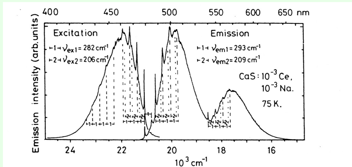
CaS:CeのPLスペクトルおよびPL励起スペクトル (両者で関与するフォノンが異なることに注意)
